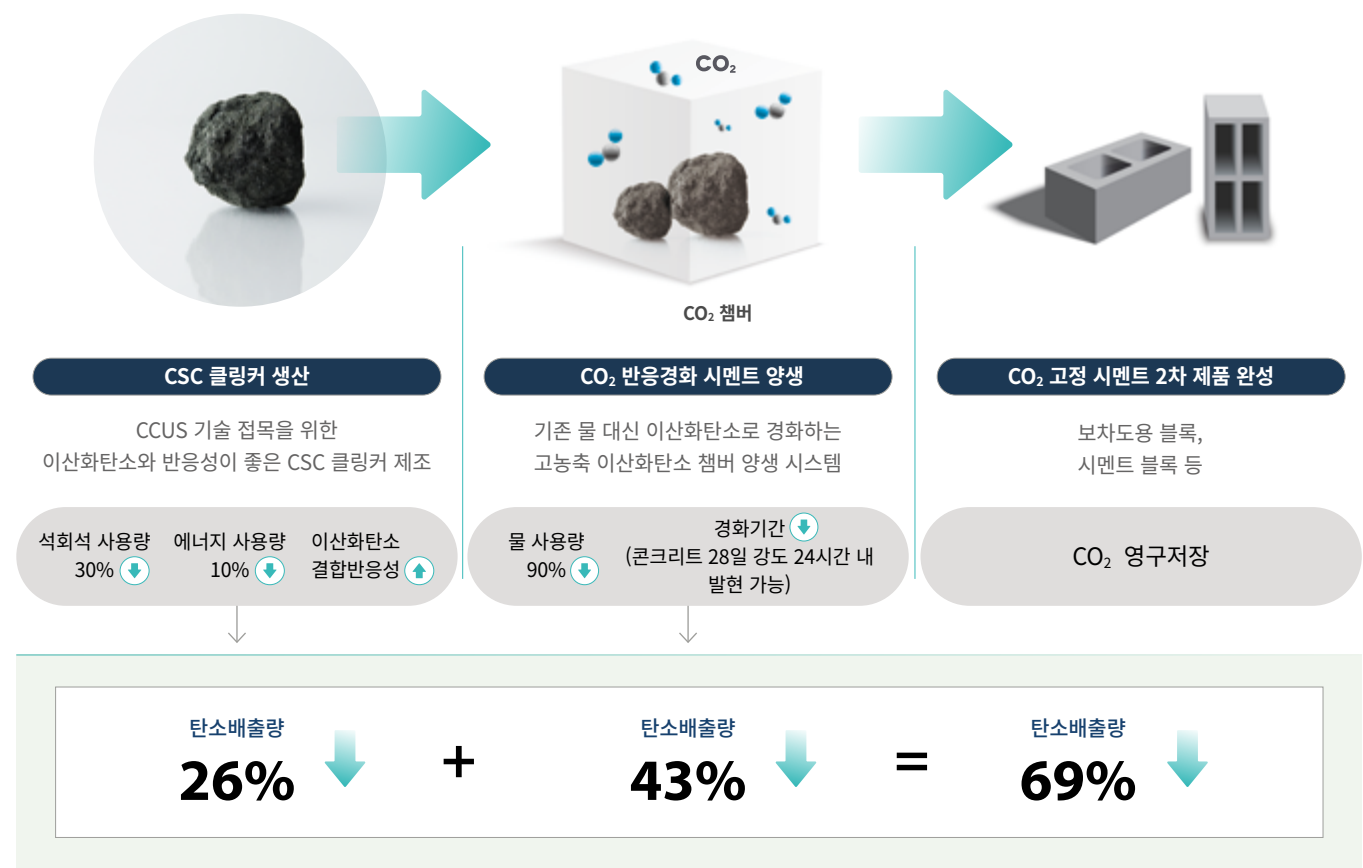
→ 이산화탄소 반응경화 시멘트 및 건설용 2차 제품 제조 기술개발 연구 구조도
